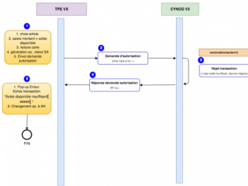
CYNOD : Traitement transaction carte ONLINE non passant solde insuffisant
